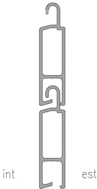
Disegno schematico fornito dal cliente
